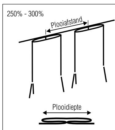
Vliesband, Enkele Platte Plooi
