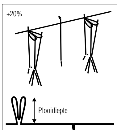
Vliesband, . . . . . plooi met Retourplooi
