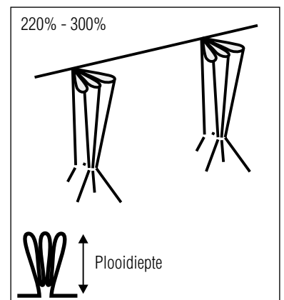
Vliesband, Triplooi
